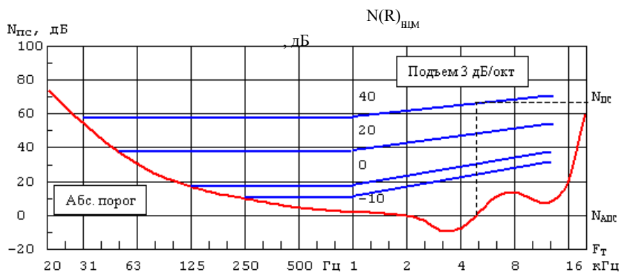
Рис.10. Кривые порога слышимости тона F_T при маскировке белым шумом
